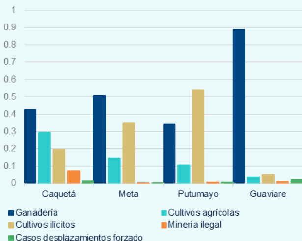
Gráfico B3. IMPORTANCIA DE LAS VARIABLES PARA LOS DEPARTAMENTOS DEL ARCO AMAZÓNICO
