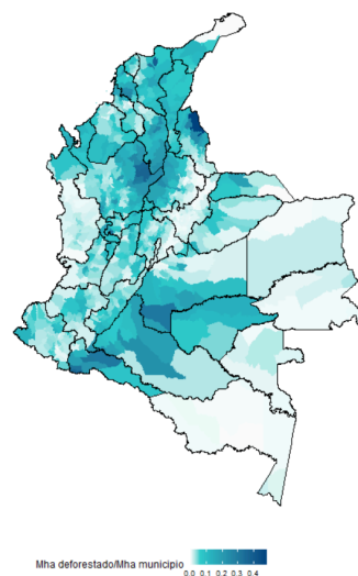
Gráfico 6. PÉRDIDA DE COBERTURA ARBÓREA ACUMULADA MUNICIPAL, 2001-2023 (MHA)
